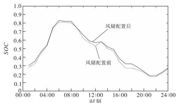
图9 风储配置前后的SOC变化趋势
