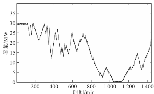
图5 安徽省网某风电场30 MW典型日出力曲线
