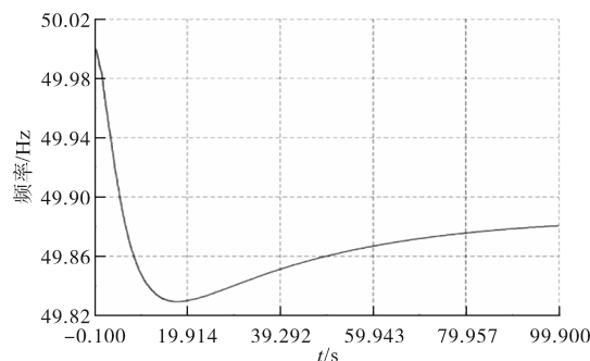
图12 配置前的频率变化
