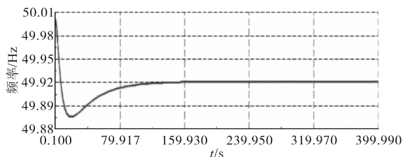
图10 仅在负荷作用下的系统频率
