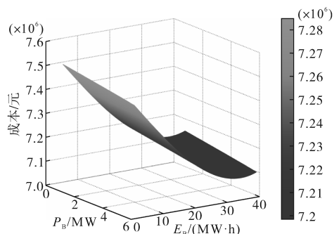
图7 成本与 P_B 和 E_B 的关系
