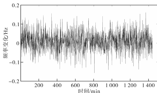
图6 安徽省网某风电场24 h频率变化
