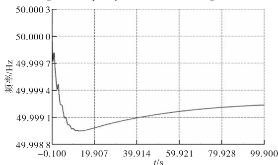
图13 风储并网后的频率变化
