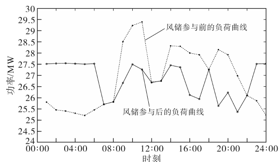
图8 风储参与前后的负荷曲线
