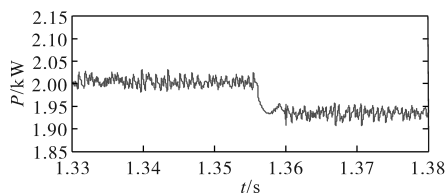
图 8 大功率变频器系统降额运行观测图
