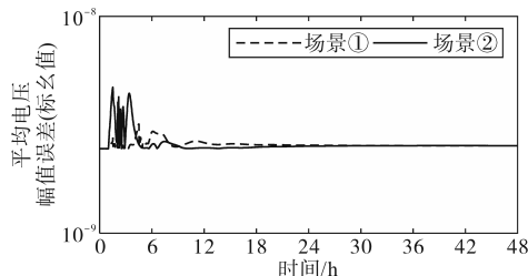
图18 算例2平均电压幅值误差
