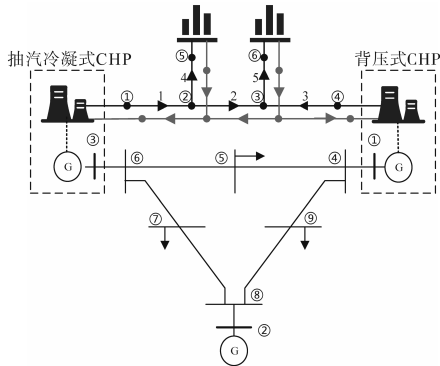
图2 算例1测试系统拓扑结构示意图
