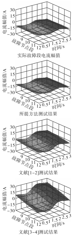
图3 不同故障辨识方法的电流幅值检测结果 Fig.3 Current amplitude detection results of different
